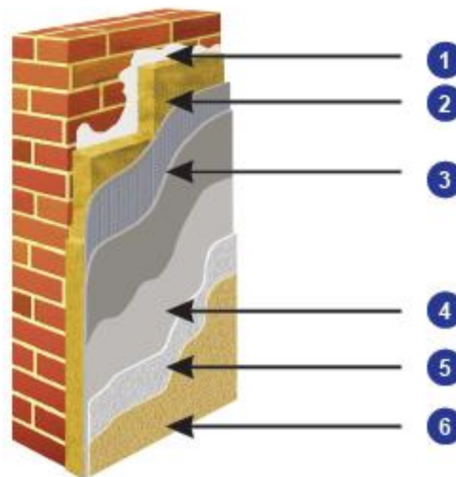
Fasadni sistem sa pločama od kamene vune
