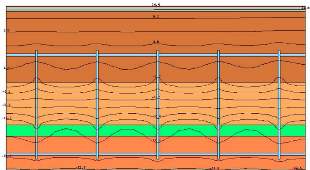
Горизонтальный разрез
