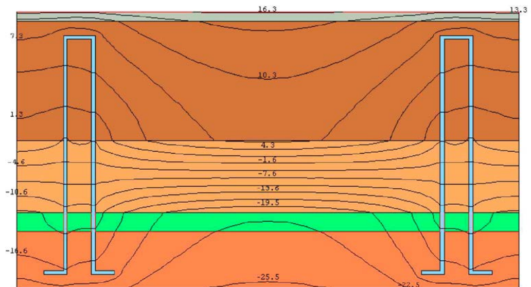
Горизонтальный разрез
