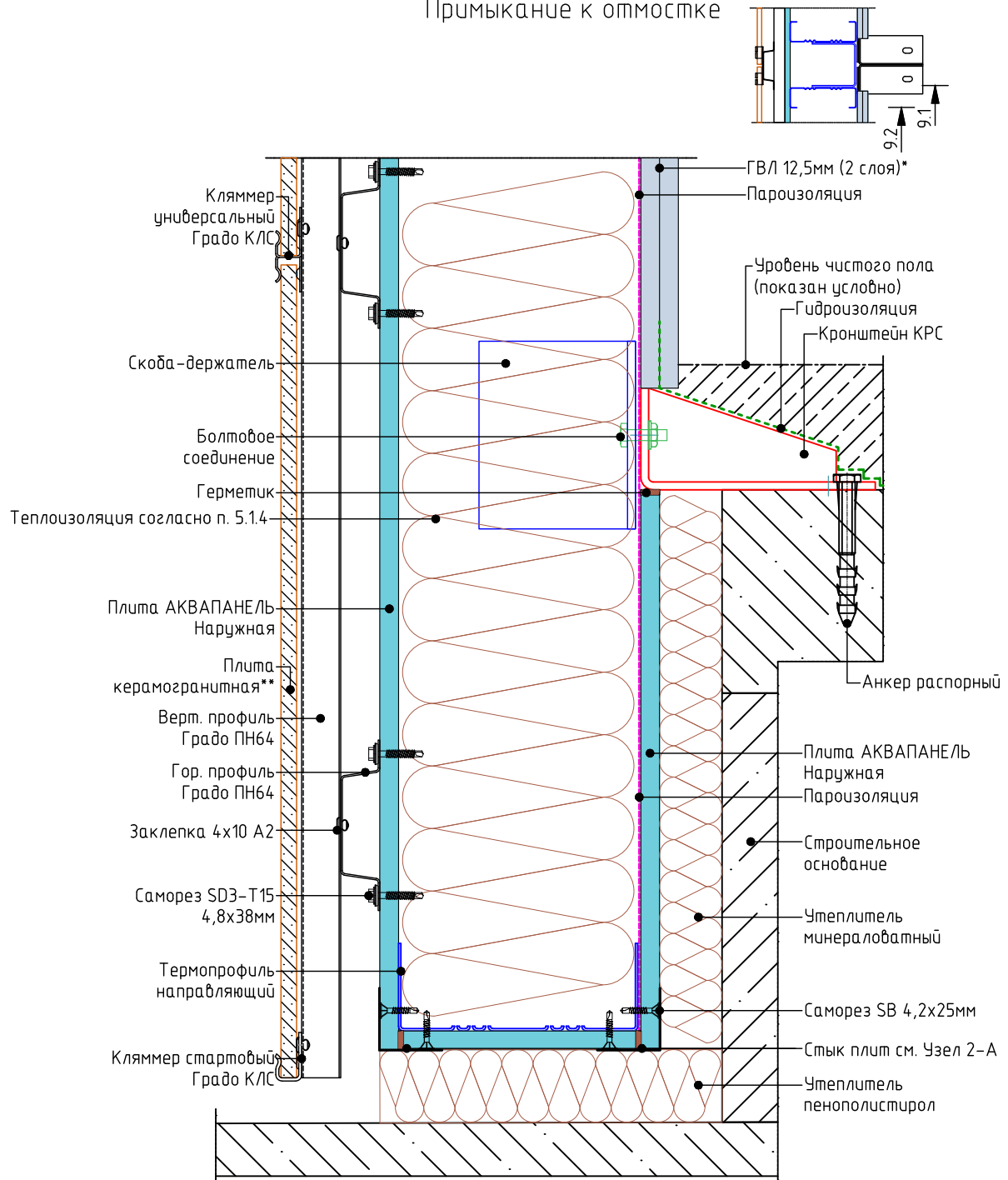
Узел 9.1. Вертикальный разрез стартового модуля Примыкание к откоске
