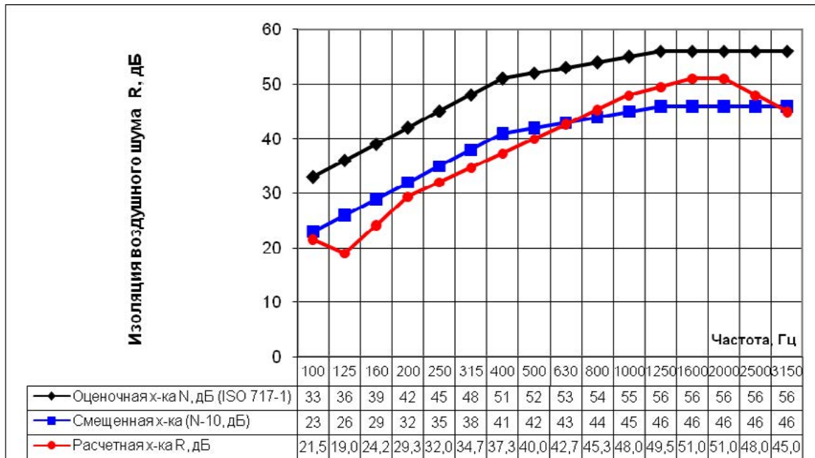
Рисунок В.2. Определение индекса звукоизоляции каркасной перегородки с заполнением звукопоглощающим материалом
