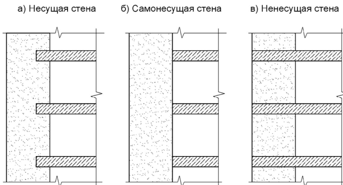
Рисунок 4.1. Схематические решения наружных стен
