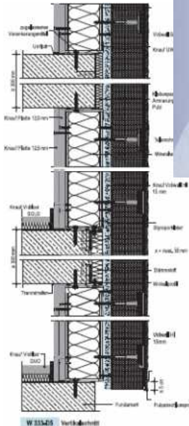
Knauf nevetreni fasadni sklop
