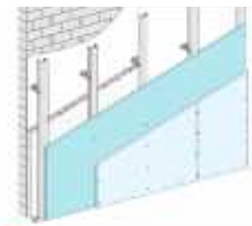
ikay W123P1 Perspektiv Vertikal
