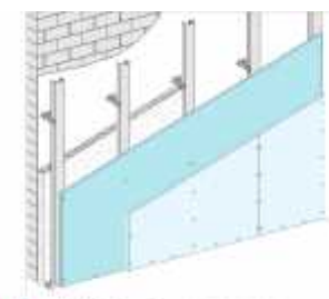
knauf W623-P1 Perspektiv: Konstruktions
