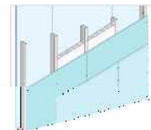
knauf W124-P1 Pano: Knauf Akustik
