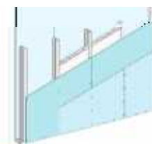
Knauf W112P1 Perspektiv Metallboden
