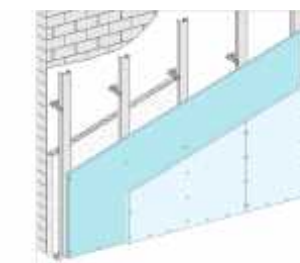
knauf W623-P1 Perspektiv: Konstruktions
