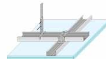
knauf D112-P1 Pano: Grund-Träger Aluminium
